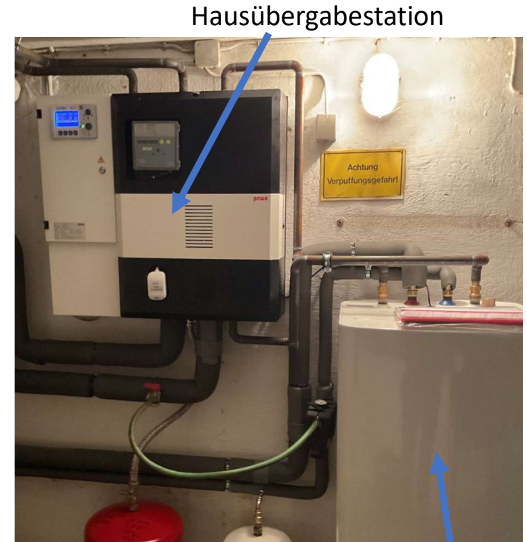
WW-Speicher (145 l)
